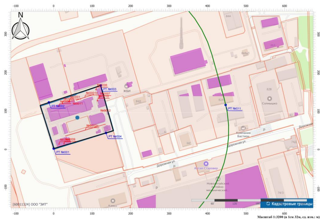
Рис. 5.14. Расположение контрольного поста (PT №011)
