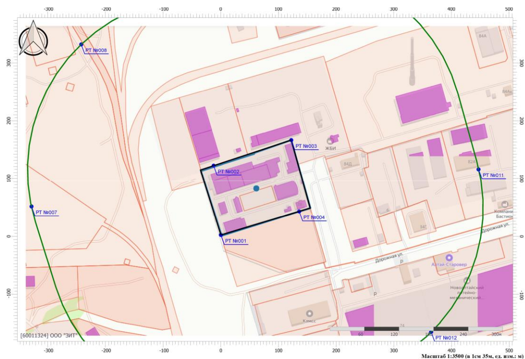
Рис. 3.12. Карта-схема расположения расчетных точек (РТ)
