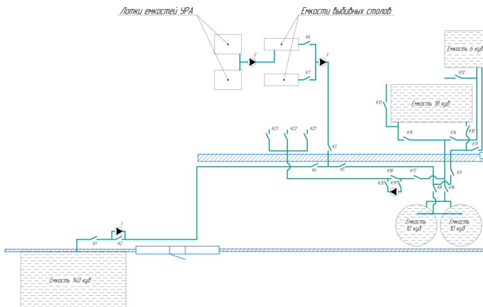
Рис. 1.3. Схема сбора электролита сернокислотного
