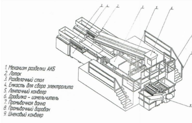
Рис. 1.2. Линия разделки АКБ «ИвТарЛони»
