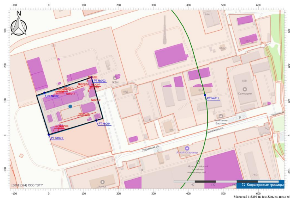
Рис. 5.15. Расположение контрольного поста (PT №011)
